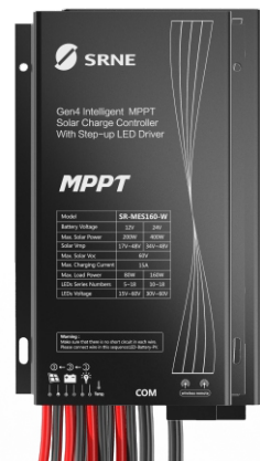
SR-MES160-R/W
