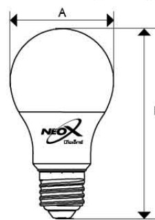
Dimension (mm.)
